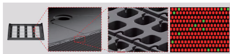
図1. QuantStudio MAP16 Digital PCRプレートの拡大図
